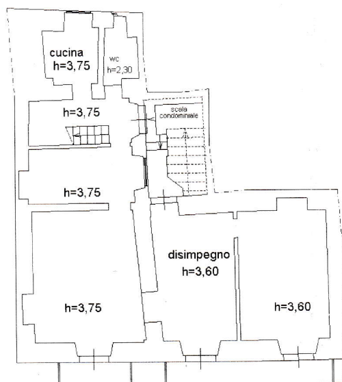
PRIMO PIANO
